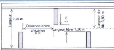
Schéma « type » et exemples d'aménagement d'un dispositif de chicanes de ralentissement
